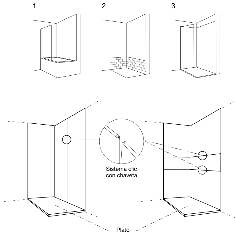
Instalación en horizontal
