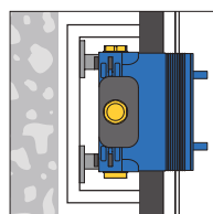
Installation devant le mur : montage sur supports dans un coffrage
