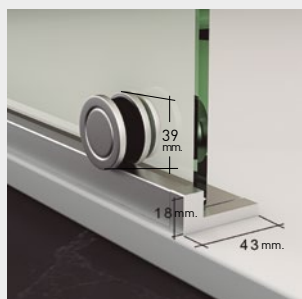
Perfil inferior + rodamiento.
