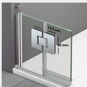
Bisagra doble + junquillo de estanqueidad.
