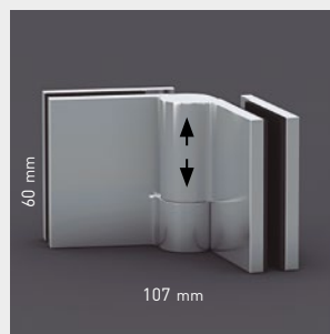
Bisagra vidrio-vidrio replegable 180° exterior. Elevable 3mm.
