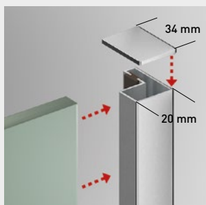
Cerco a pared, cierre sin goma magnética.
