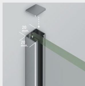
Cerco a pared U-20, vidrio fijo.
