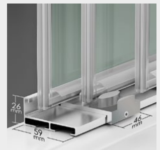
Perfil inferior 3P + guía base deslizante.
