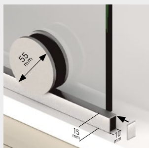
Rodamiento + Sección perfil inferior.
