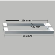
Detalle tirador H, para anchos > 75 cm.
