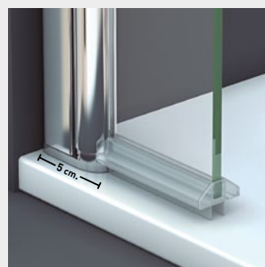
Vierteaguas con doble goma. Modelo Sport.
