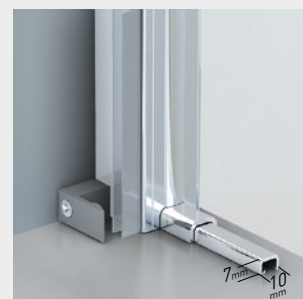
Detalle tope de cierre + perfil inferior.
