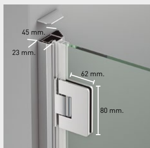
Bisagra rotativa 180°. Apertura 90°+90°.
