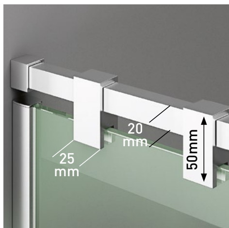
Detalle barra de sujeción horizontal 180°.
