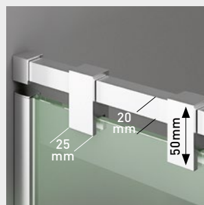
Detalle soporte de barra 180°
