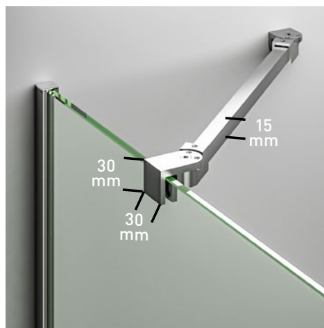
Brazo de sujeción 45° - Articulada.
