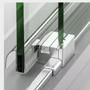
Liberación de puertas. Perfil de estanqueidad 7x10 mm.
