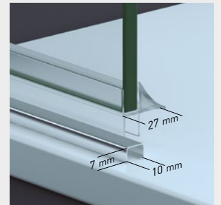
Perfil de estanqueidad + vierteaguas doble ala.
