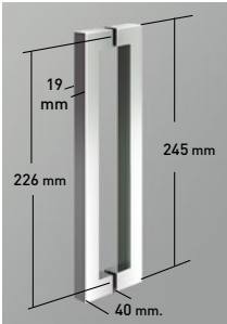
Detalle de tirador.
