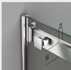
Soporte a pared (vista exterior). Puerta 8mm + cierre magnético.
