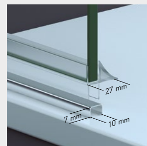
Perfil de estanqueidad + vierteaguas doble ala.
