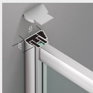
Cerco a pared + Compensador UL-25 modelo CP. Corrige desnivel de paredes. Perfilería aluminio.
