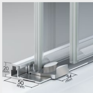
Perfil inferior 2P + guía base deslizante.
