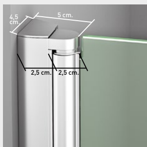
Cerco a pared + eje de giro 180°.
