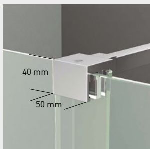
Brazo de sujeción estándar.
