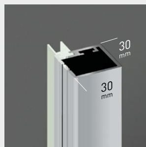
Sección perfil a pared + goma de cierre.
