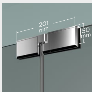
Detalle bisagra doble
