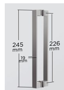
Detalle de tirador.
