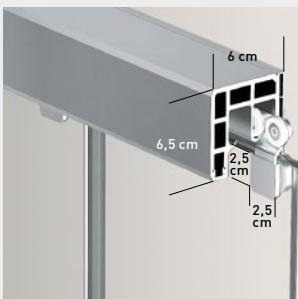
Cerco 2P, vista exterior. Soporte rodamiento semioculto.
