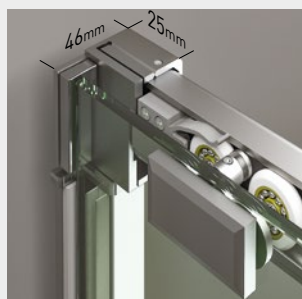
Tope fin de carrera. Vista interior.
