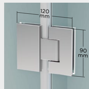
Detalle de bisagra vidrio-vidrio Acero Inoxidable
