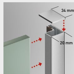
Cerco a pared. Puerta sin goma magnética.
