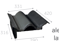
Teja de alero remate lateral izqdo
