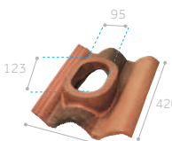
Teja con salida circular
