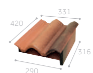
Teja de alero remate lateral dcho
