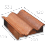
Teja de alero remate lateral izqdo
