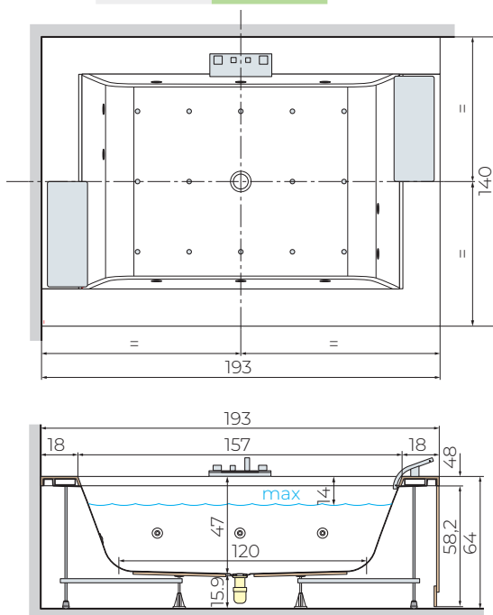
BLANCO BRILLO
