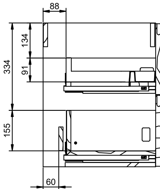
B-B ( 1 : 8 )
